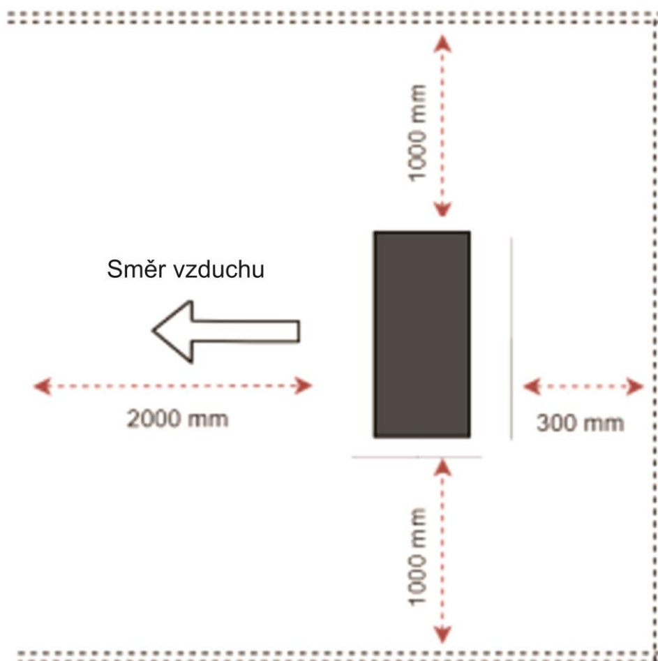
Obrázek 10: Minimální vůle
