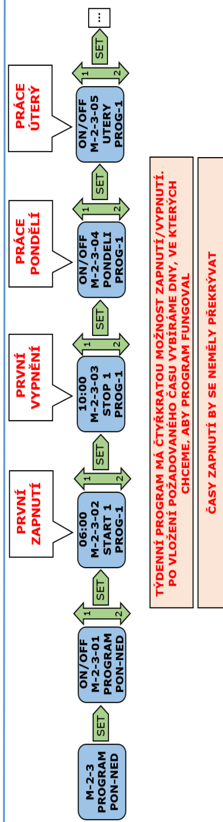
Vývojový diagram 3.
